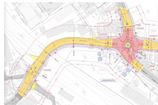
Situationsplan Laupenstrasse, Wald: Neubau Kreisel und Ergänzung Velowege
